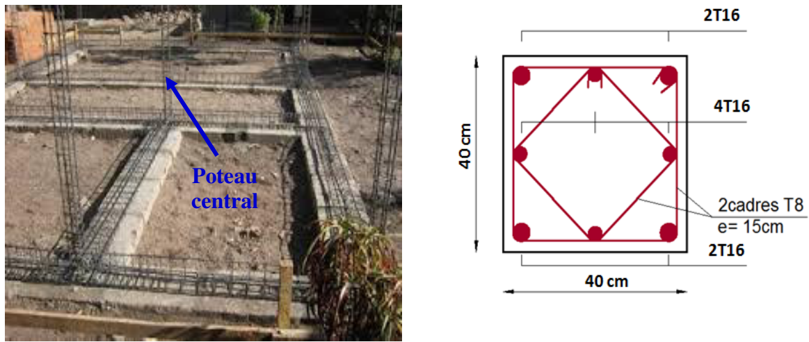
Figure VI.13 : Disposition du ferrailage du poteau central.
